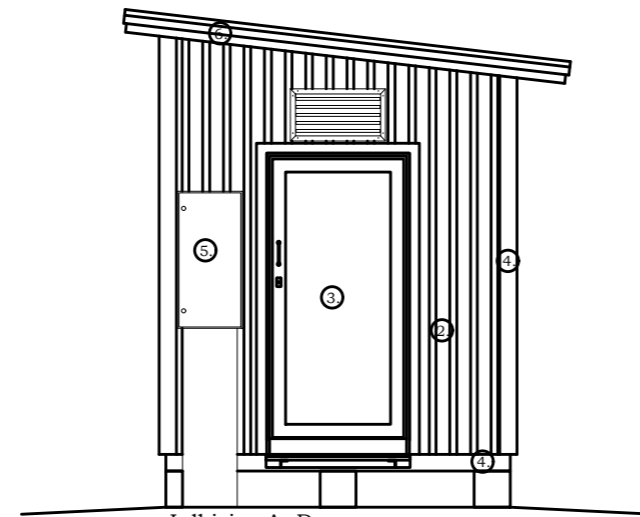
Julkisivu A.-D.
